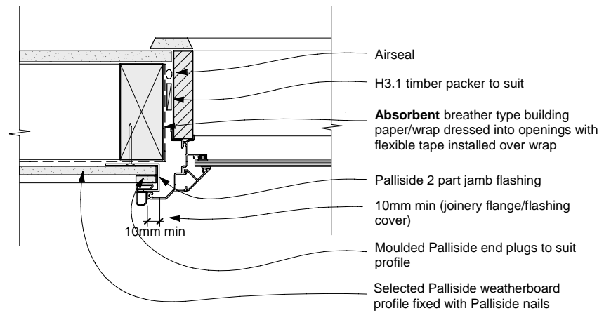
DF03 Window Jamb
